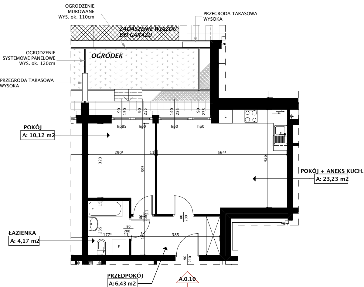
ZESPÓŁ BUDYNKÓW MIESZKALNYCH Z USŁUGAMI TOWARZYSZĄCYMI Poznań, ul. Morzyczńska
