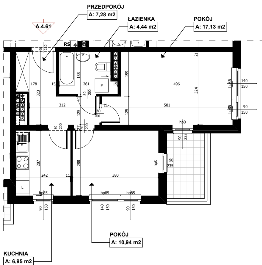
ZESPÓŁ BUDYNKÓW MIESZKALNYCH Z USŁUGAMI TOWARZYSZĄCYMI Poznań, ul. Morzycańska
