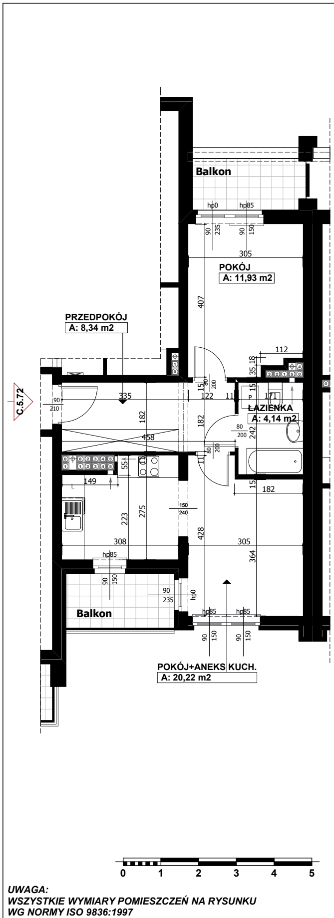
ZESPÓŁ BUDYNKÓW MIESZKALNYCH Z USŁUGAMI TOWARZYSZĄCYMI Poznań, ul. Morzycznańska
